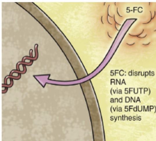
Figura 10. Mecanismul de acțiune al flucitozinei (25)
