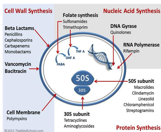
Figura 2. Mecanismele de acțiune ale antibioticelor
