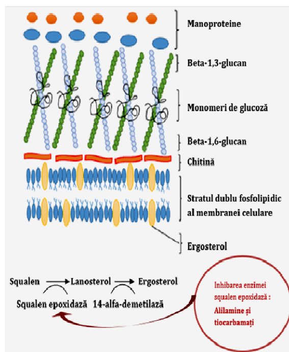
Figura 9. Mecanismul de acțiune al terbinafinei (26)
