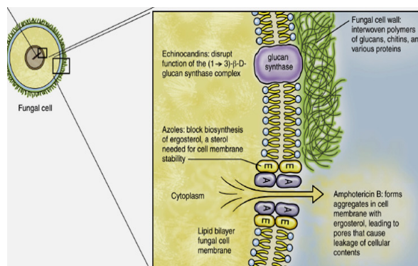
Figura 6. Mecanismul de acțiune al Amfotericinei B (25)
